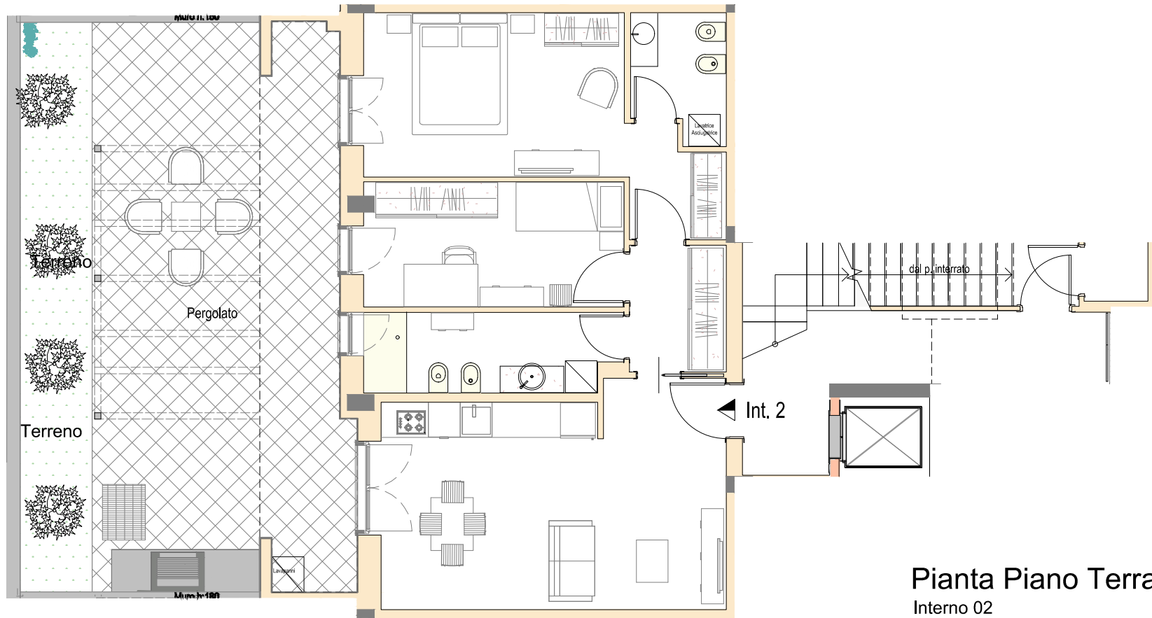
SCHEMA GRAFICO SUPERFICI E PERTINENZE - INTERNO 2
